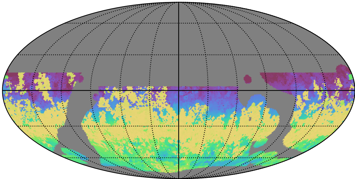
weather_cloudso0v3.5_10yrs WFD r band: AngleRange rotSkyPos
