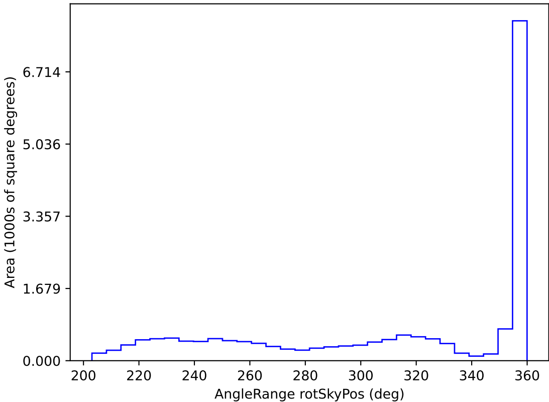
weather_cloudso0v3.5_10yrs WFD r band: AngleRange rotSkyPos
