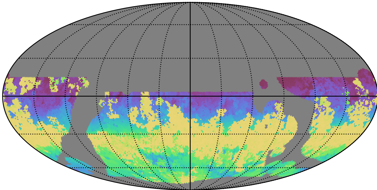
weather_cloudso0v3.5_10yrs WFD i band: AngleRange rotSkyPos
