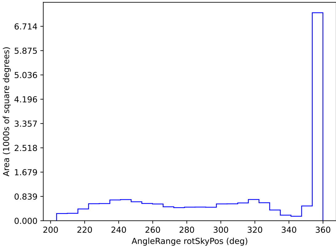
weather_cloudso0v3.5_10yrs WFD i band: AngleRange rotSkyPos
