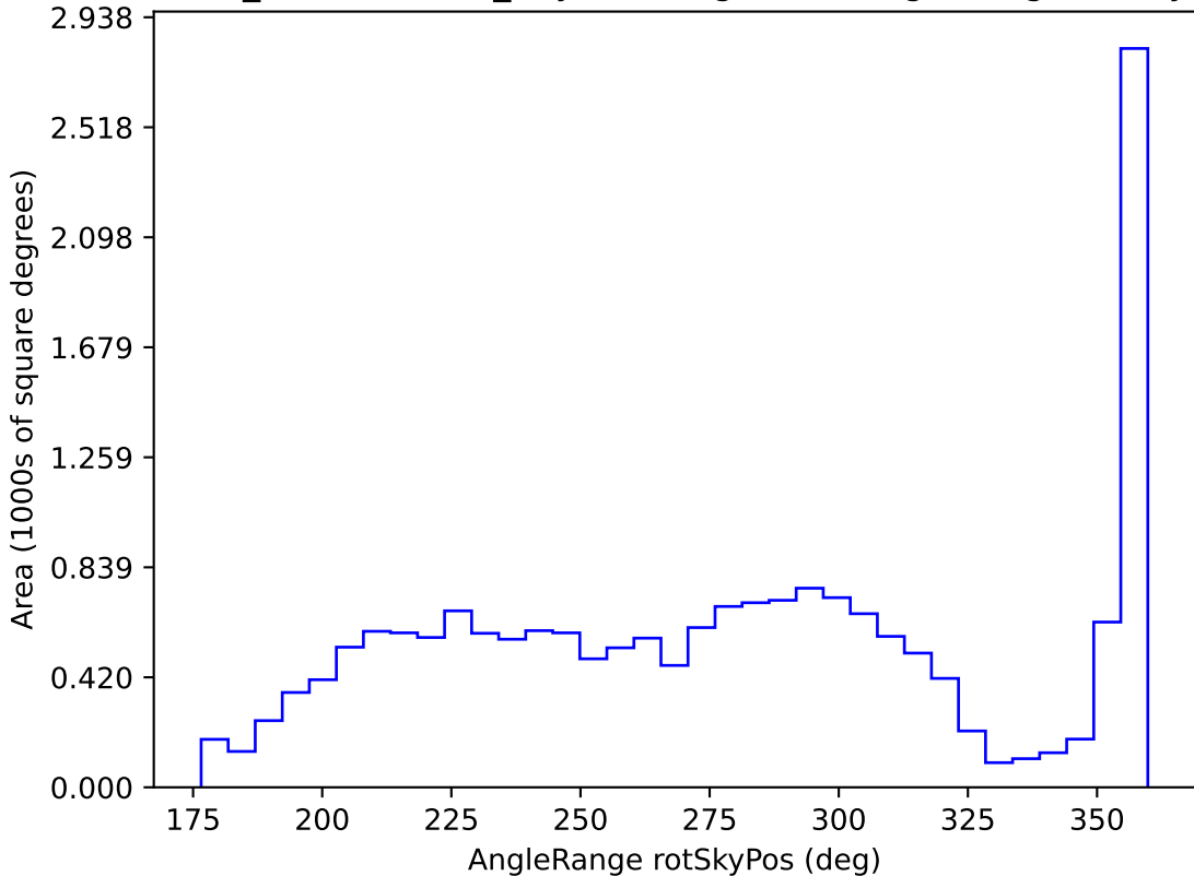
weather_cloudso0v3.5_10yrs WFD g band: AngleRange rotSkyPos
