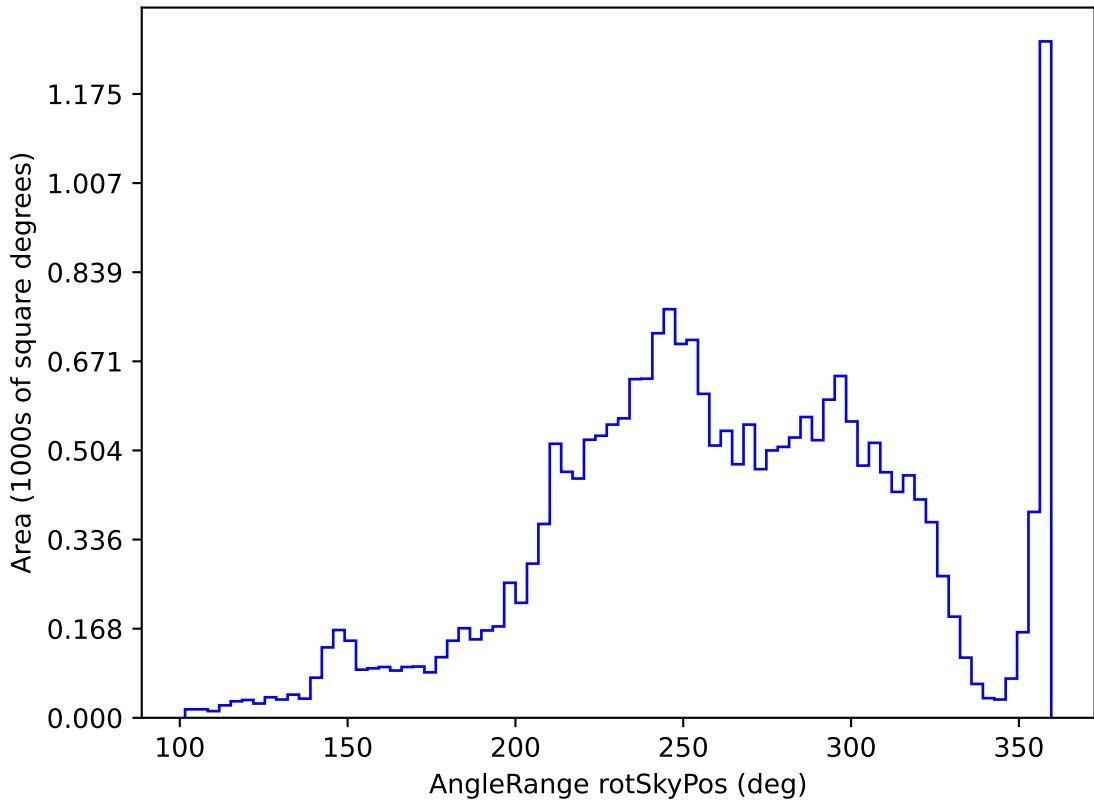
weather_cloudso0v3.5_10yrs All sky y band: AngleRange rotSkyPos
