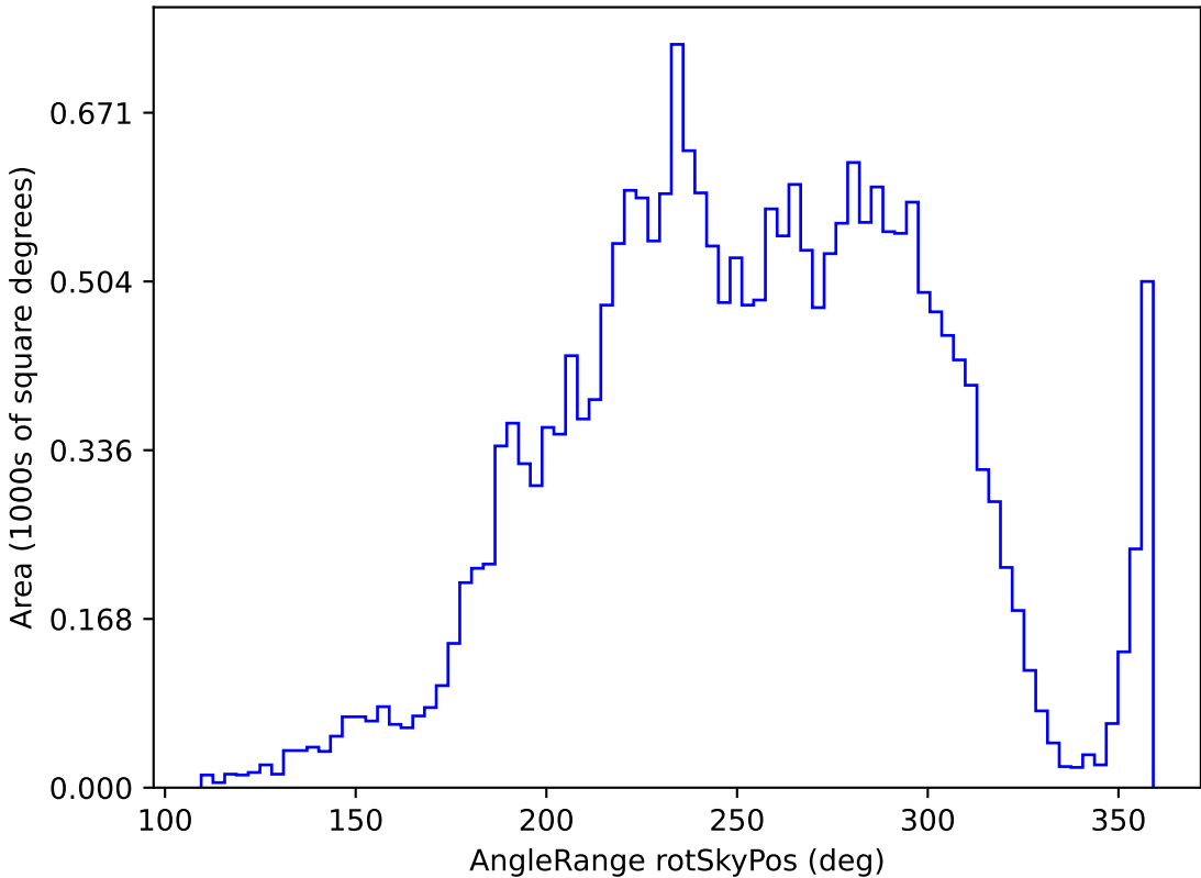
weather_cloudso0v3.5_10yrs All sky u band: AngleRange rotSkyPos
