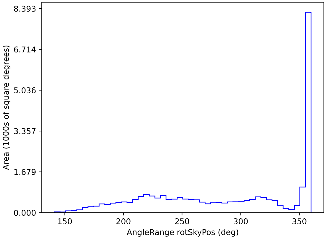
weather_cloudso0v3.5_10yrs All sky r band: AngleRange rotSkyPos
