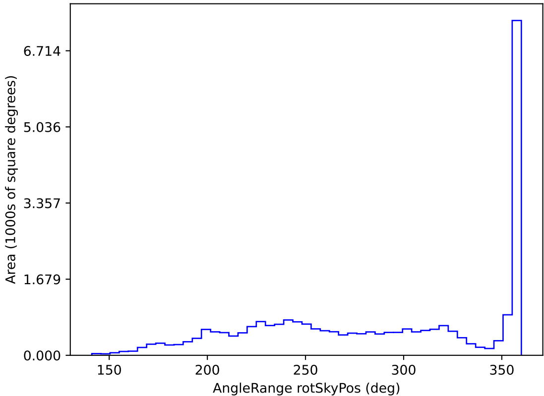
weather_cloudso0v3.5_10yrs All sky i band: AngleRange rotSkyPos
