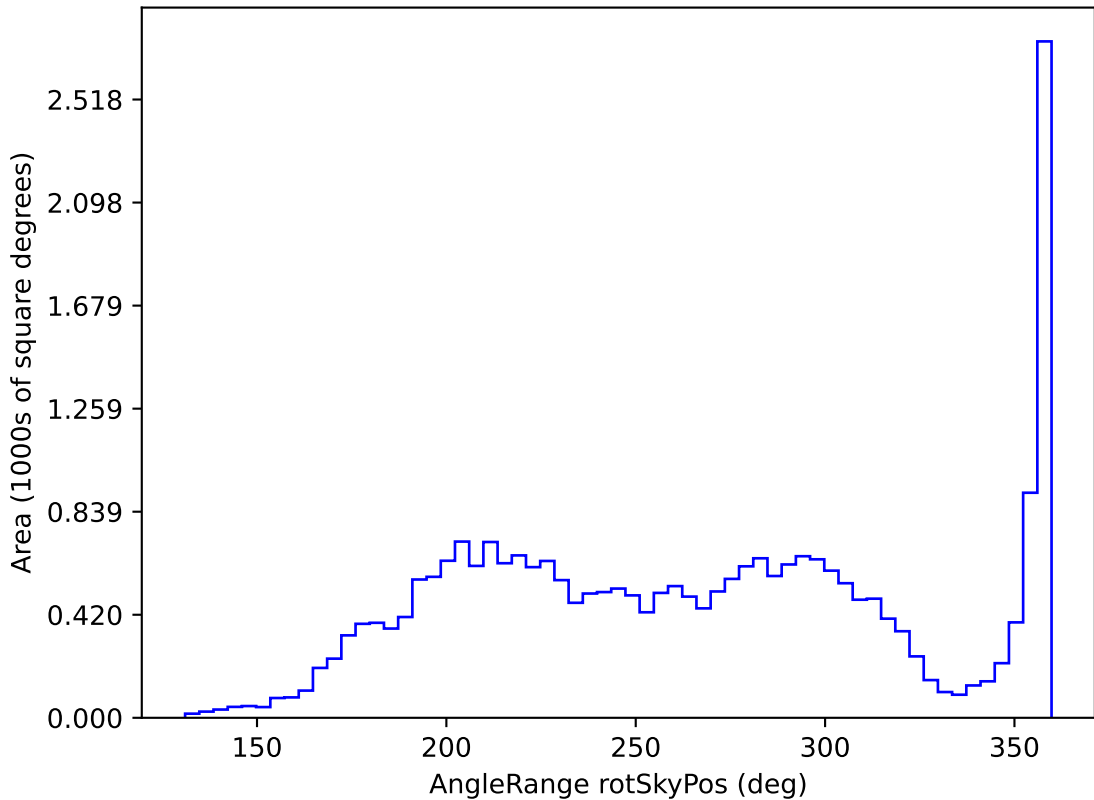
weather_cloudso0v3.5_10yrs All sky g band: AngleRange rotSkyPos
