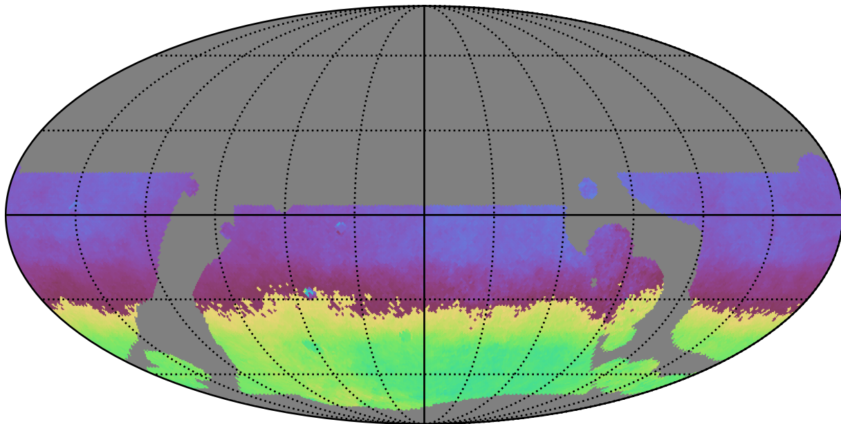
weather_cloudso0v3.5_10yrs WFD y band: AngleMean rotSkyPos
