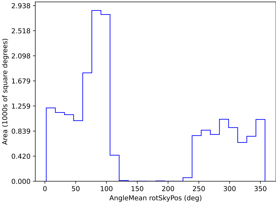
weather_cloudso0v3.5_10yrs WFD y band: AngleMean rotSkyPos
