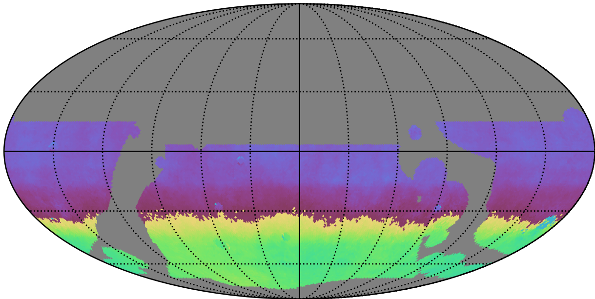
weather_cloudso0v3.5_10yrs WFD i band: AngleMean rotSkyPos
