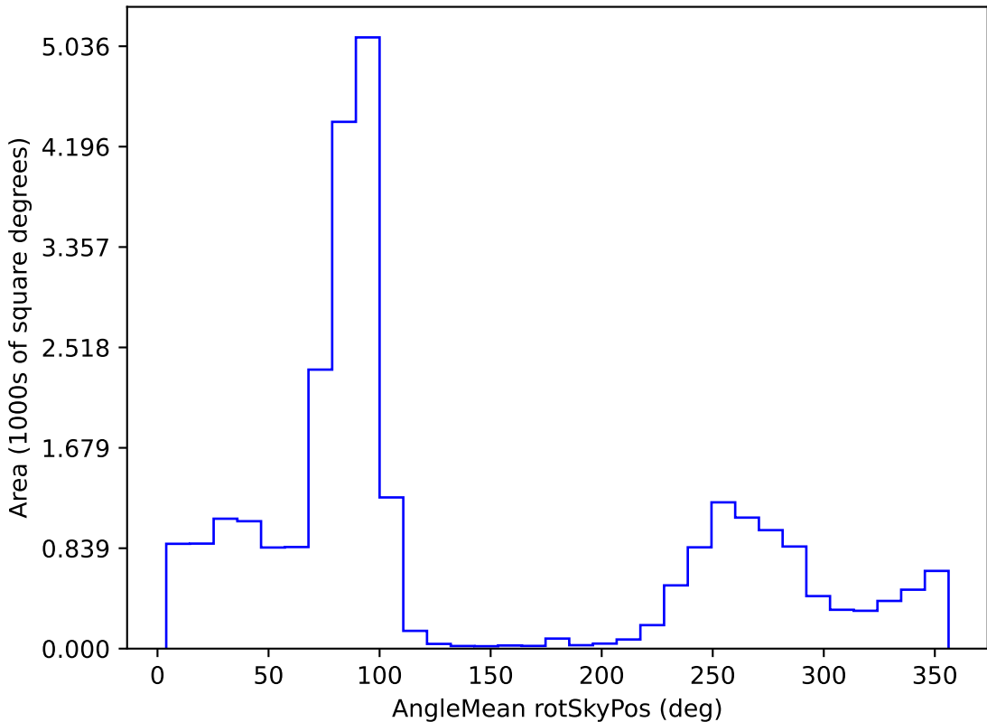
weather_cloudso0v3.5_10yrs All sky i band: AngleMean rotSkyPos
