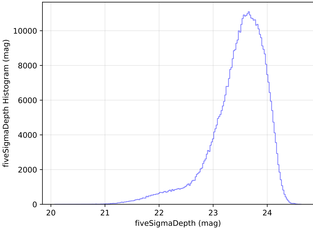
weather_cloudso0v3.4_10yrs i: fiveSigmaDepth Histogram
