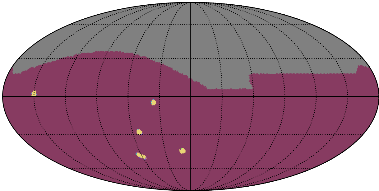
weather_cloudso0v3.4_10yrs : NumberOfQuickRevisits
