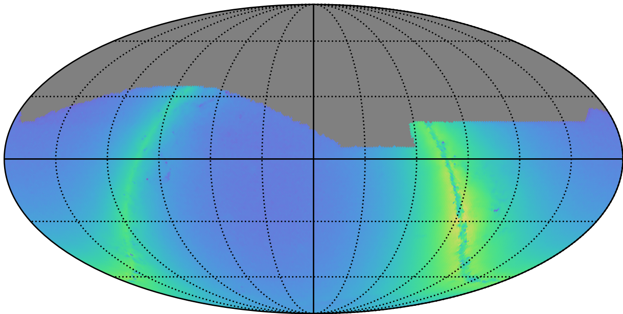
weather_cloudso0v3.4_10yrs r: Nstars_no_crowding
