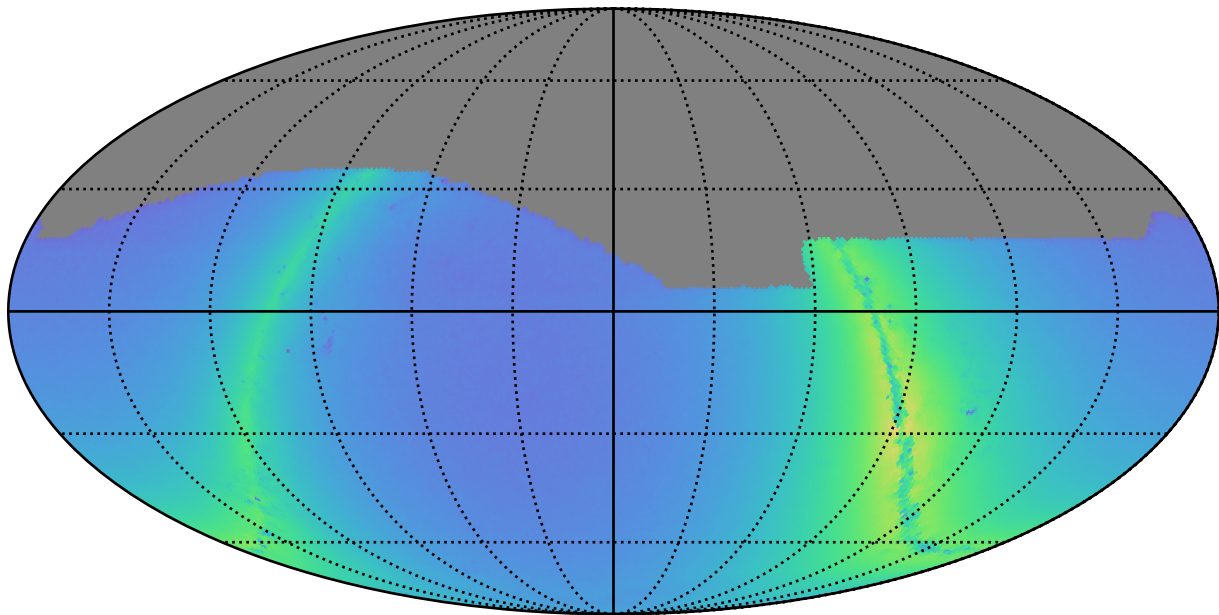
weather_cloudso0v3.4_10yrs i: Nstars_no_crowding
