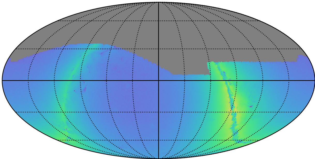
weather_cloudso0v3.4_10yrs g: Nstars_no_crowding
