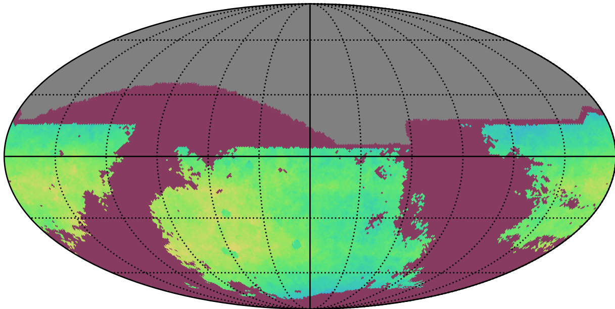
weather_cloudso0v3.4_10yrs i: NgalScale
