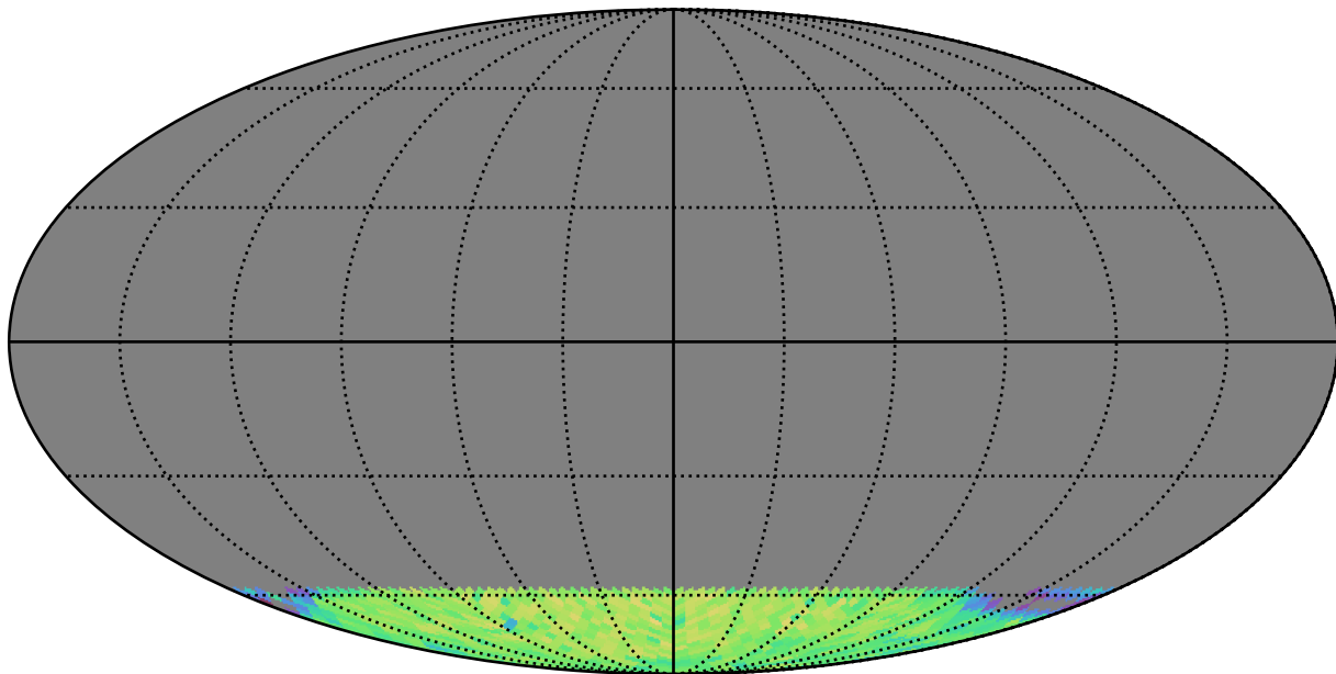
weather_cloudso0v3.4_10yrs gi SCP: LVDwarfs
