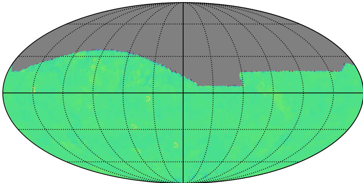
weather_cloudso0v3.4_10yrs z: Kuiper rotTelPos
