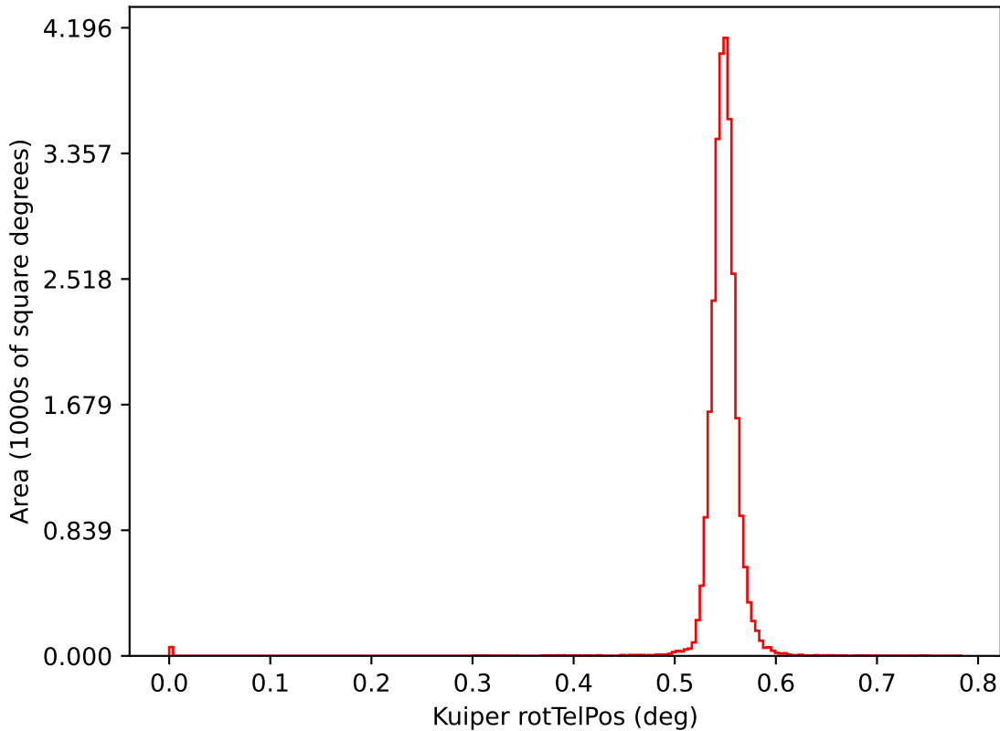
weather_cloudso0v3.4_10yrs i: Kuiper rotTelPos
