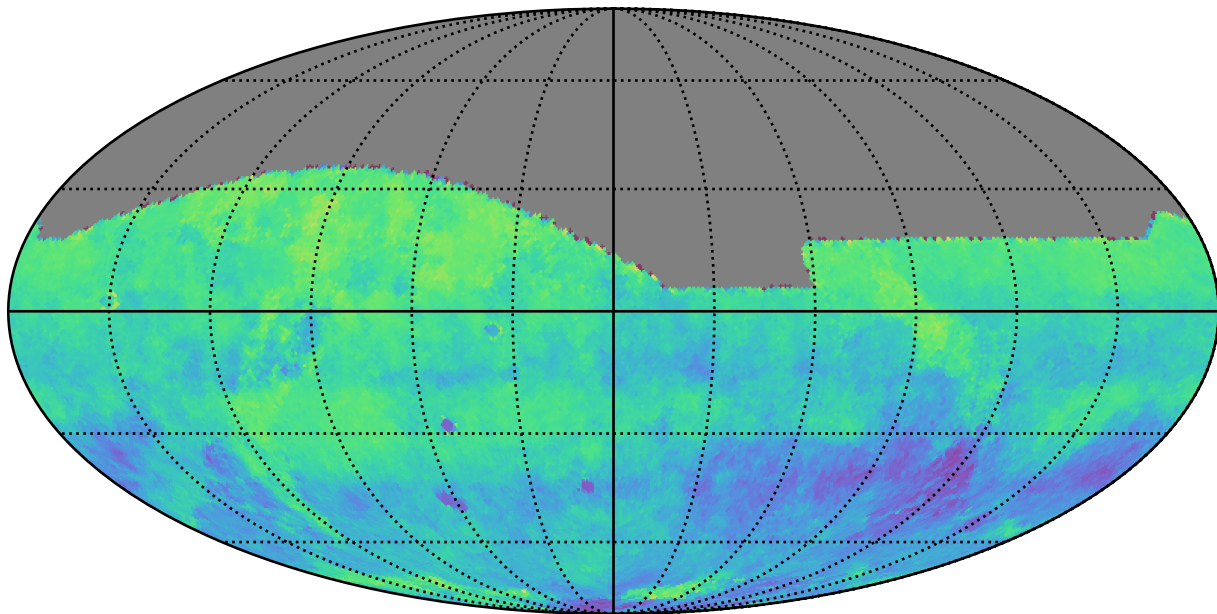
weather_cloudso0v3.4_10yrs z: Kuiper rotSkyPos
