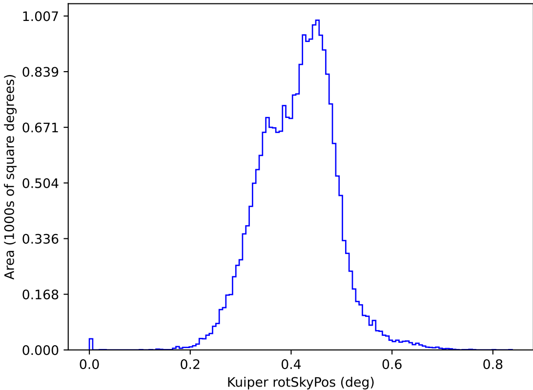
weather_cloudso0v3.4_10yrs y: Kuiper rotSkyPos
