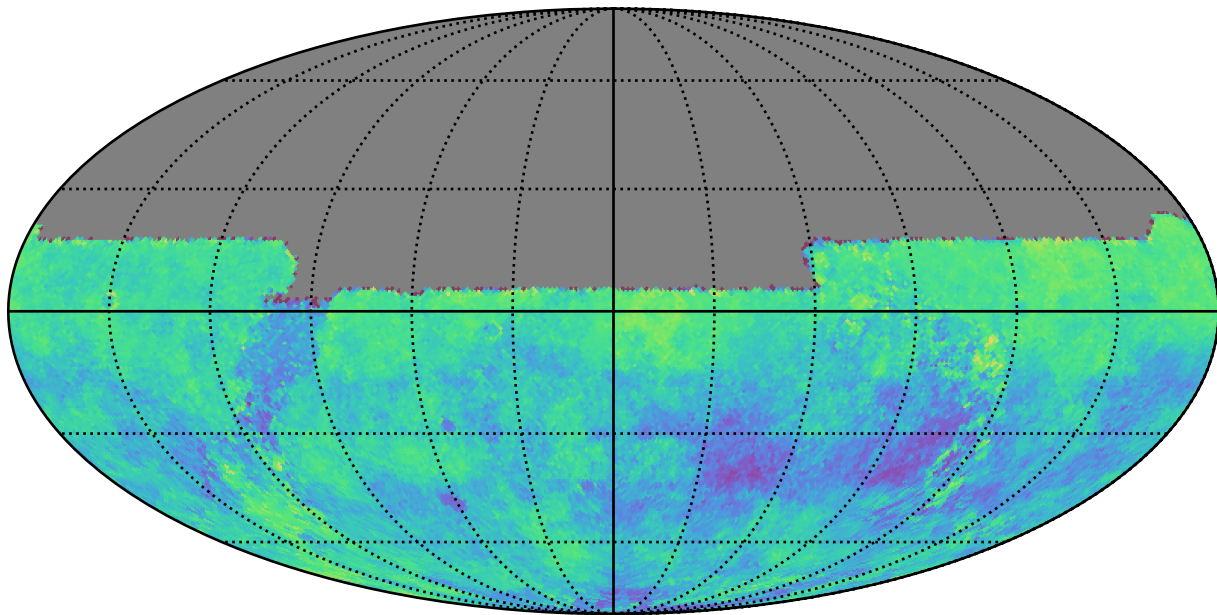
weather_cloudso0v3.4_10yrs u: Kuiper rotSkyPos
