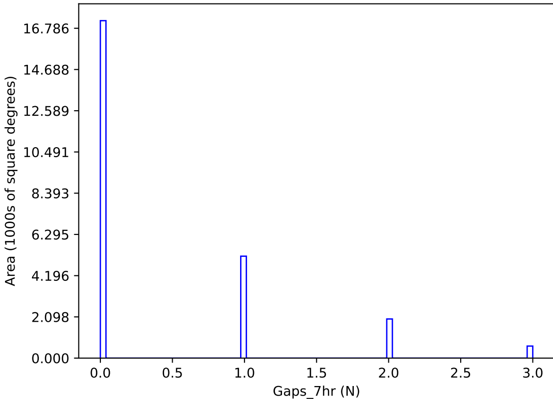
weather_cloudso0v3.4_10yrs y band: Gaps_7hr
