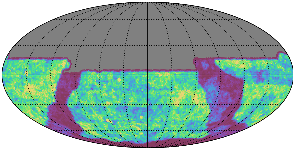
weather_cloudso0v3.4_10yrs y band: Gaps_24hr
