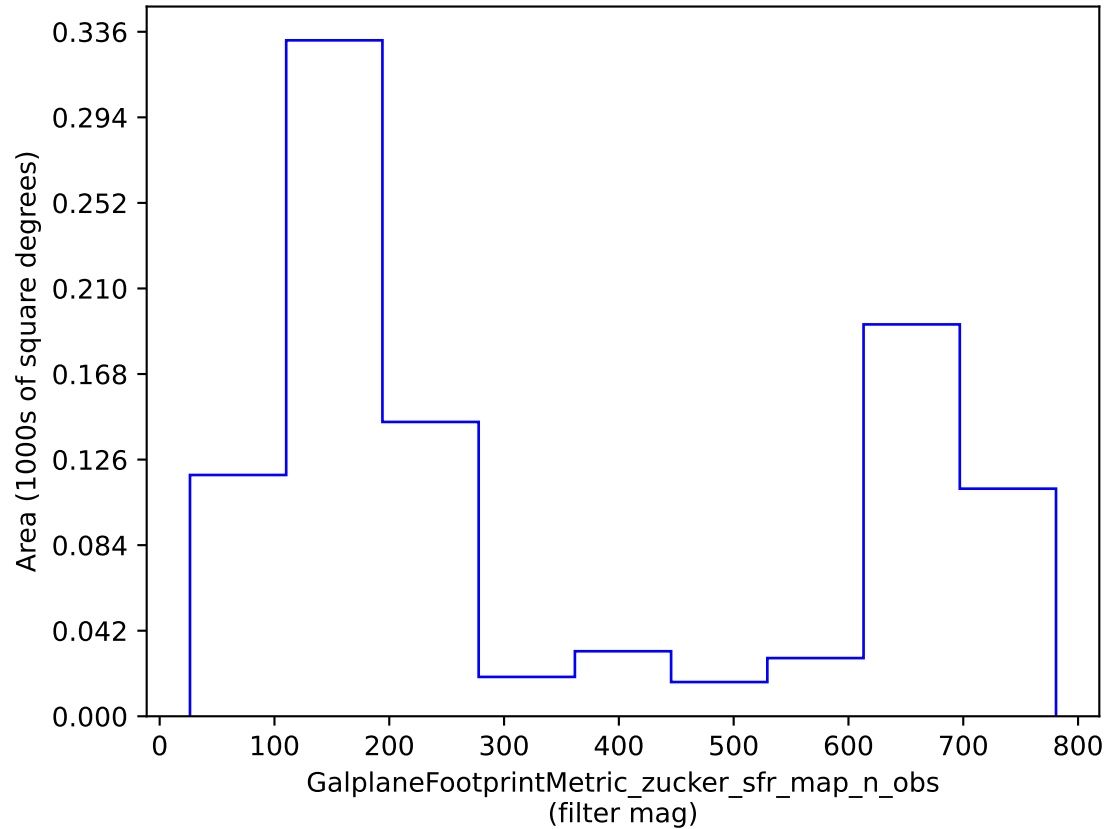
weather_cloudso0v3.4_10yrs : GalplaneFootprintMetric_zucker_sfr_map_n_obs
