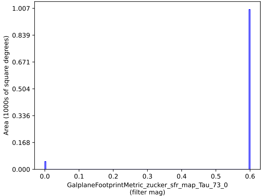
weather_cloudso0v3.4_10yrs : GalplaneFootprintMetric_zucker_sfr_map_Tau_73_0
