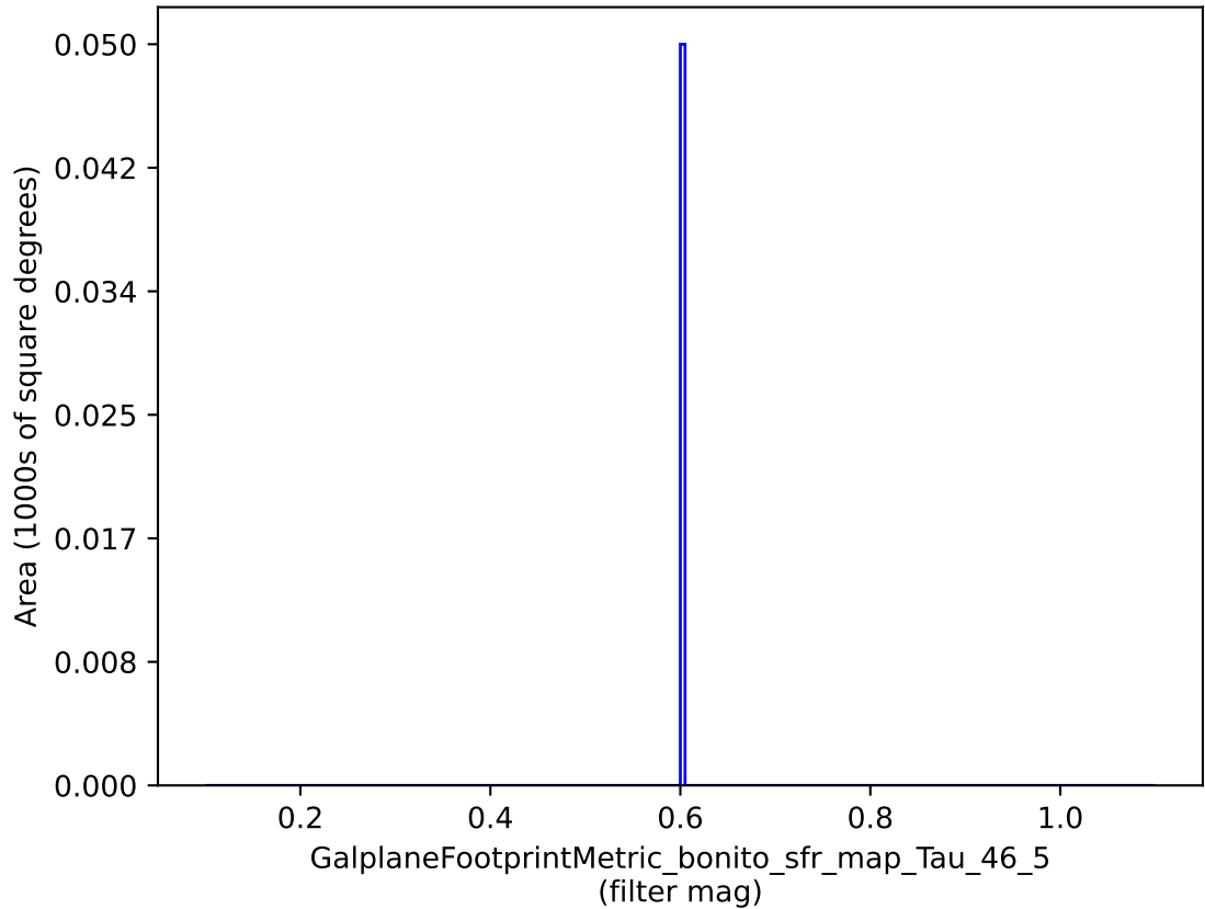
weather_cloudso0v3.4_10yrs : GalplaneFootprintMetric_bonito_sfr_map_Tau_46_5
