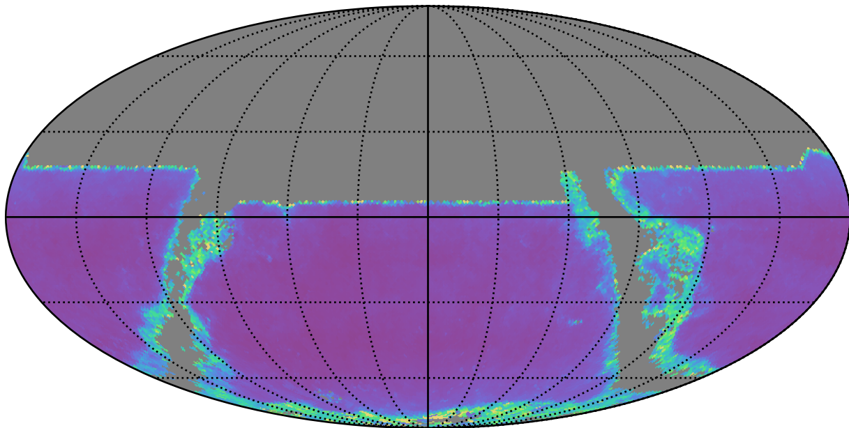
weather_cloudso0v3.4_10yrs y band: AGN SF_uncert
