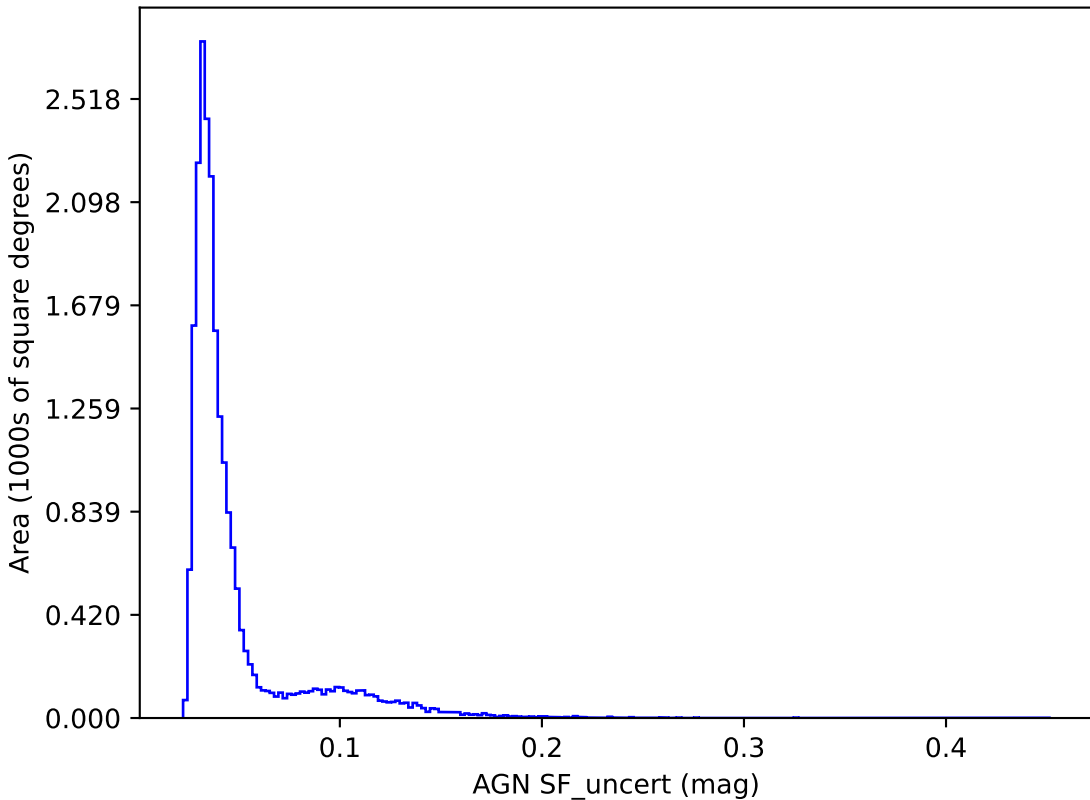
weather_cloudso0v3.4_10yrs y band: AGN SF_uncert
