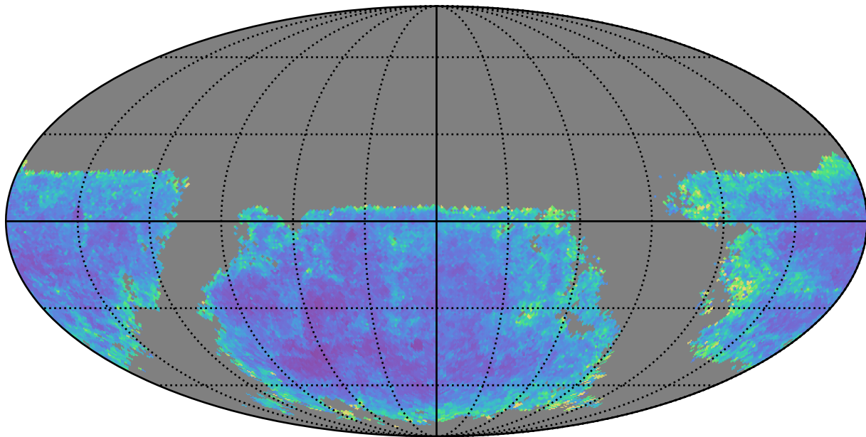
weather_cloudso0v3.4_10yrs u band: AGN SF_uncert
