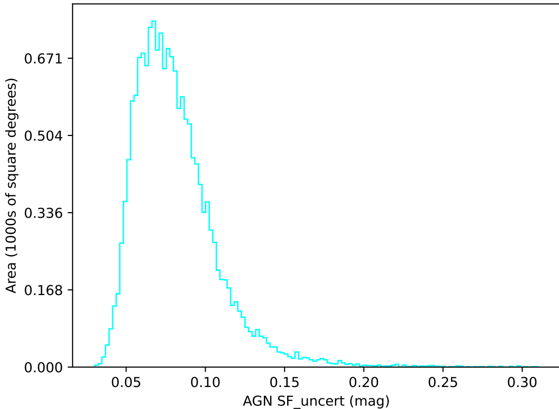
weather_cloudso0v3.4_10yrs u band: AGN SF_uncert
