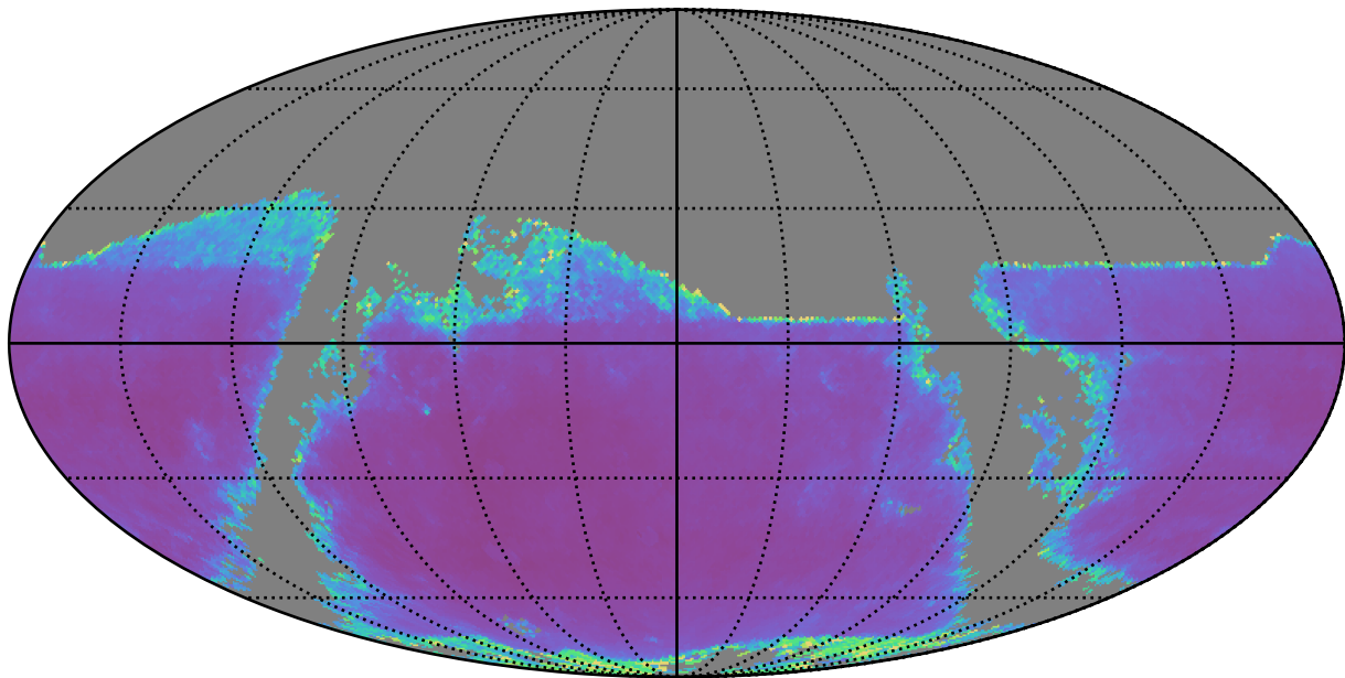
weather_cloudso0v3.4_10yrs r band: AGN SF_uncert
