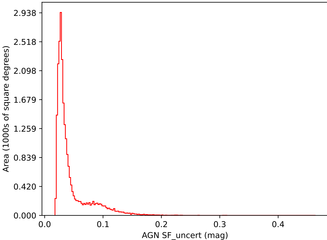
weather_cloudso0v3.4_10yrs i band: AGN SF_uncert
