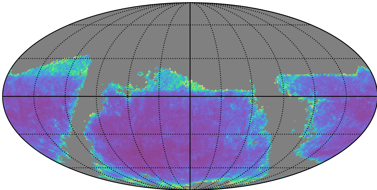
weather_cloudso0v3.4_10yrs g band: AGN SF_uncert
