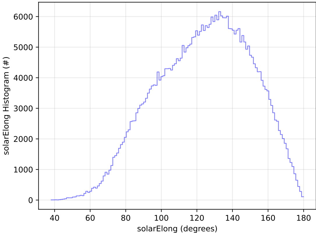
weather_cloudso0v3.4_10yrs WFD y band: solarElong Histogram
