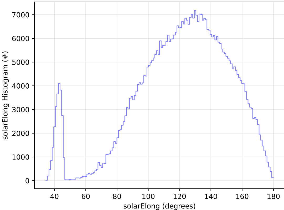
weather_cloudso0v3.4_10yrs WFD i band: solarElong Histogram
