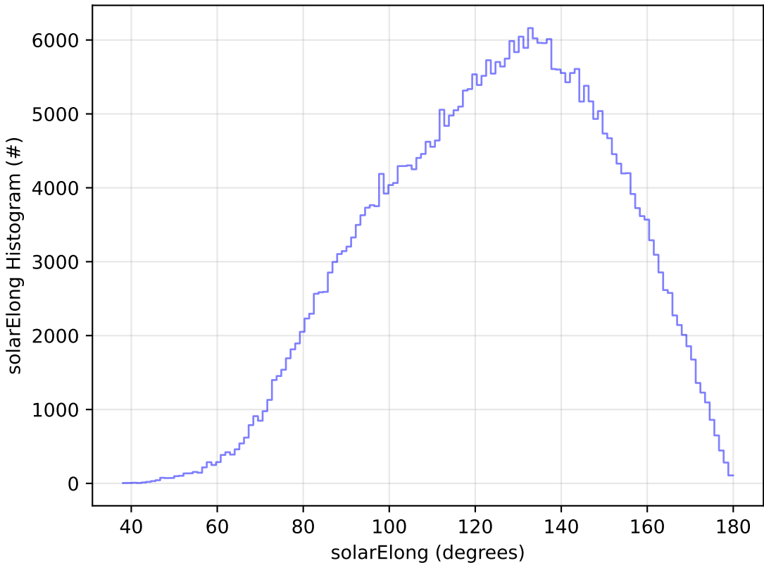
weather_cloudso0v3.4_10yrs All sky y band: solarElong Histogram
