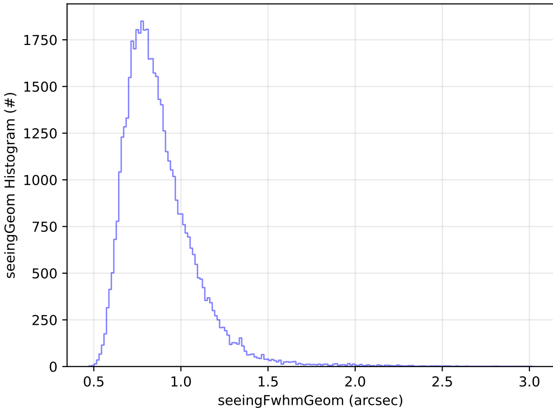
weather_cloudso0v3.4_10yrs Yr 1 y band: seeingGeom Histogram
