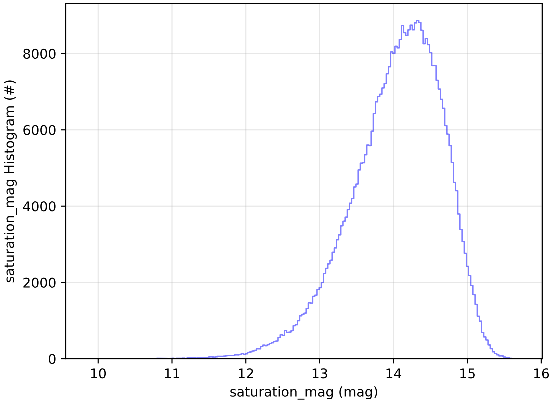
weather_cloudso0v3.4_10yrs WFD z band: saturation_mag Histogram
