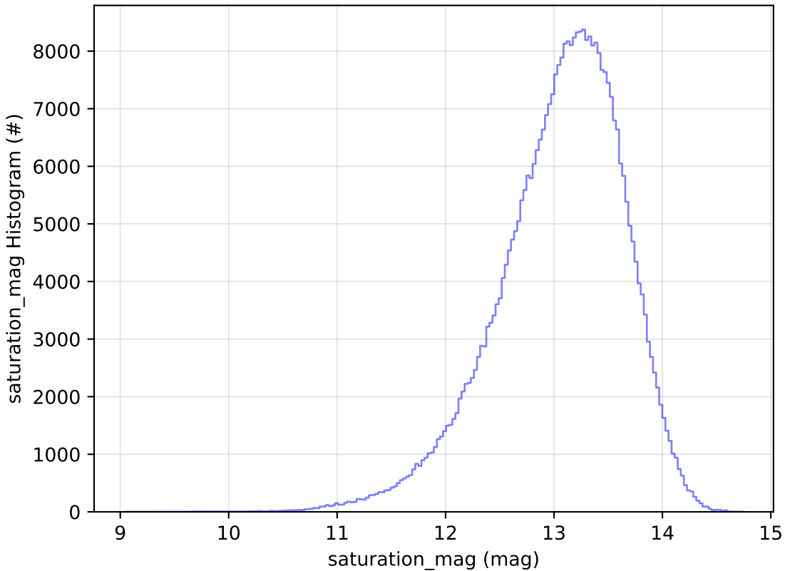
weather_cloudso0v3.4_10yrs WFD y band: saturation_mag Histogram
