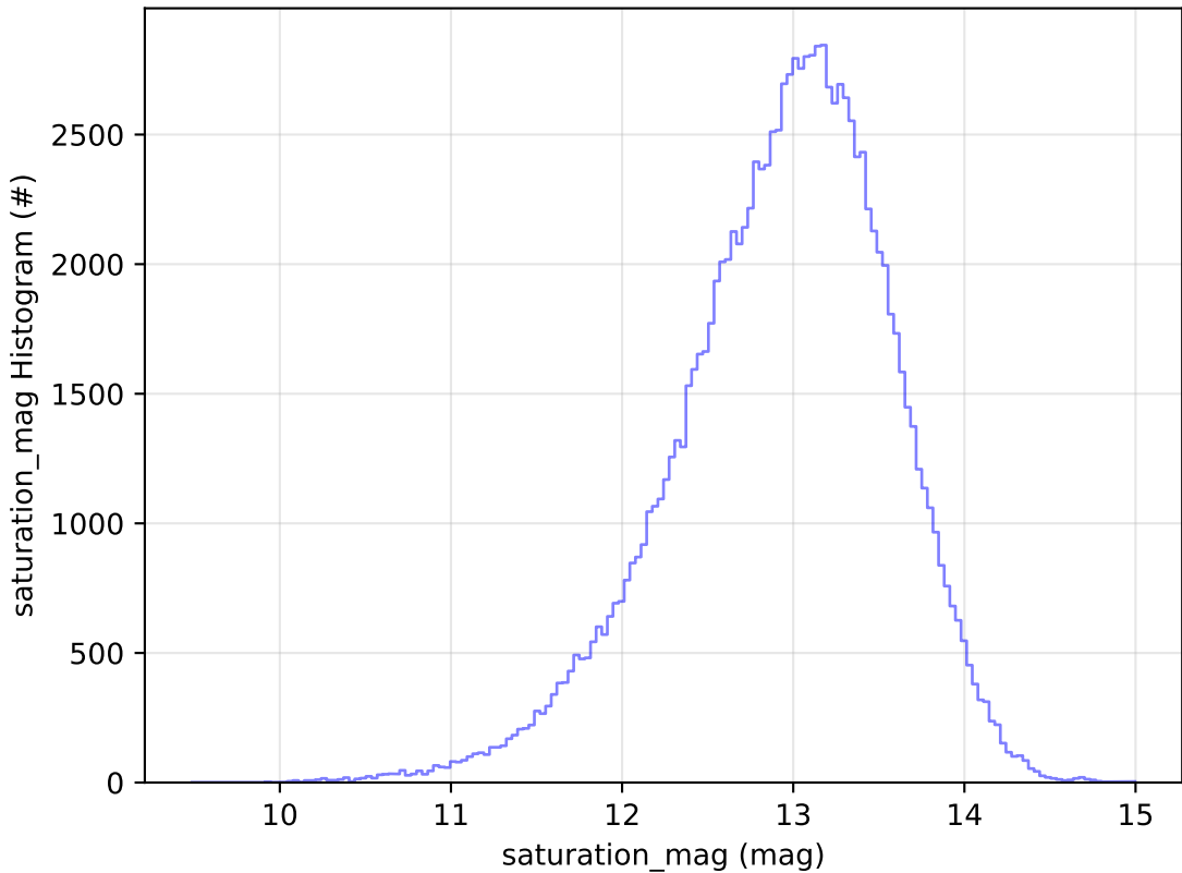
weather_cloudso0v3.4_10yrs WFD u band: saturation_mag Histogram
