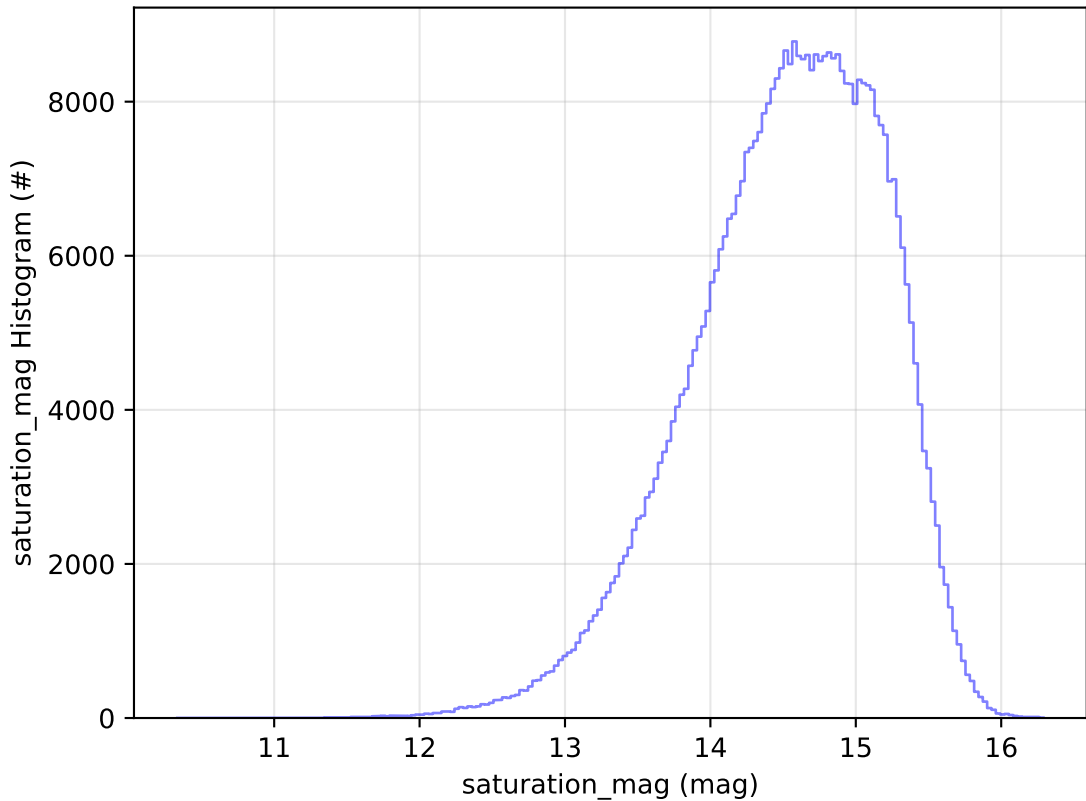
weather_cloudso0v3.4_10yrs WFD r band: saturation_mag Histogram
