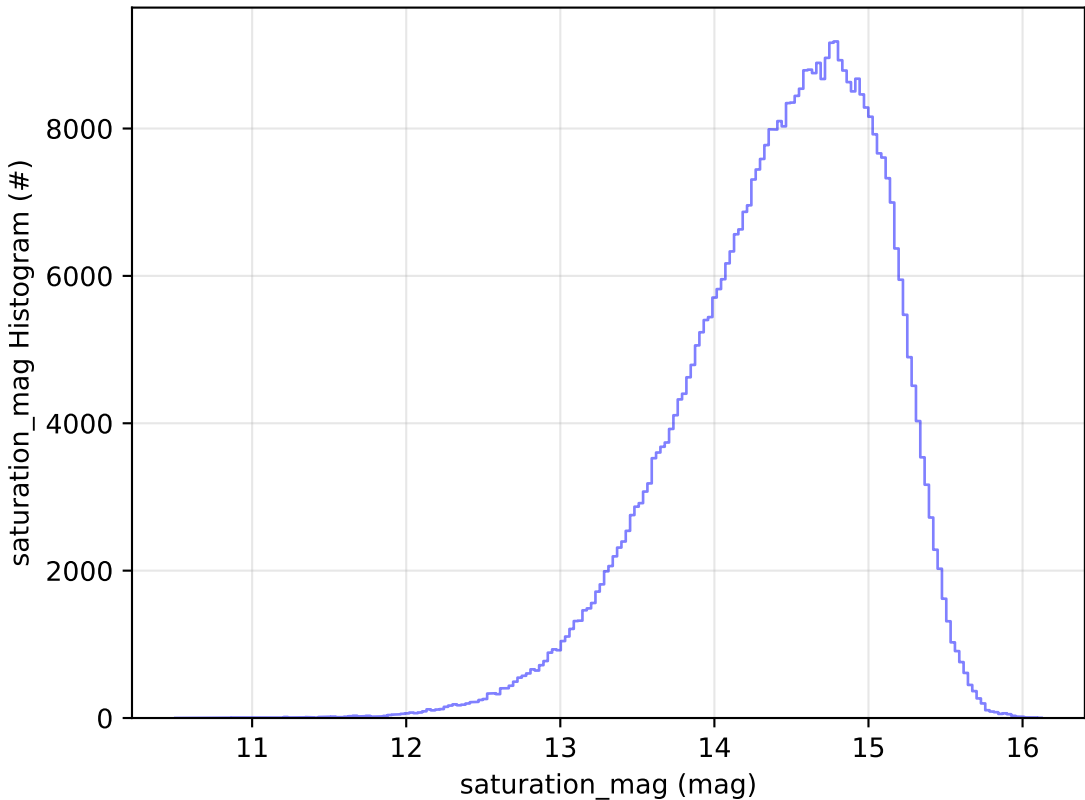
weather_cloudso0v3.4_10yrs WFD i band: saturation_mag Histogram
