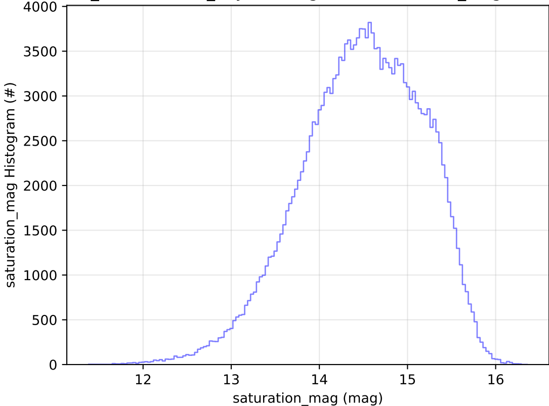
weather_cloudso0v3.4_10yrs WFD g band: saturation_mag Histogram
