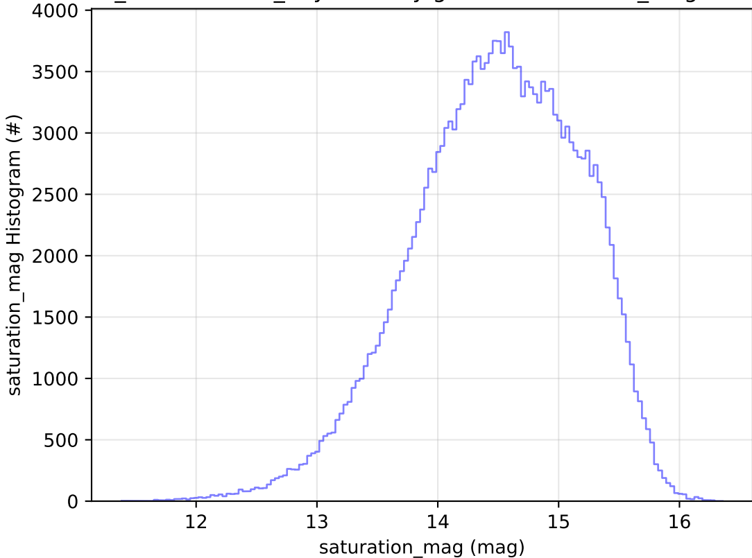
weather_cloudso0v3.4_10yrs All sky g band: saturation_mag Histogram
