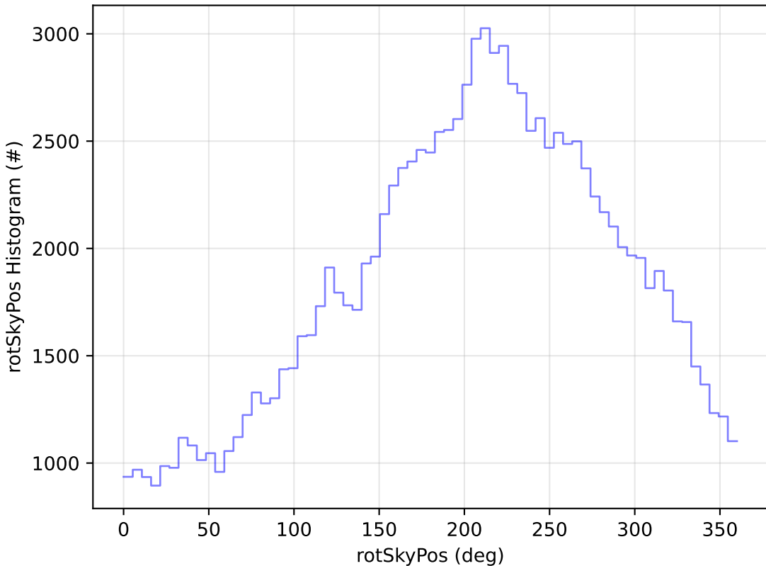
weather_cloudso0v3.4_10yrs WFD u band: rotSkyPos Histogram
